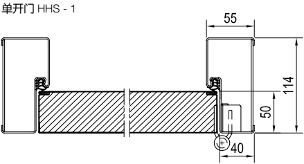
横剖视图
