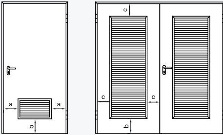
钢质通风百页 (适用于多用途门 HHS)
