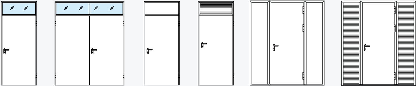
上亮 / 上楣板 / 钢质上百页 / 侧楣板 / 钢质侧百页 * (适用于多用途门 HHS)
